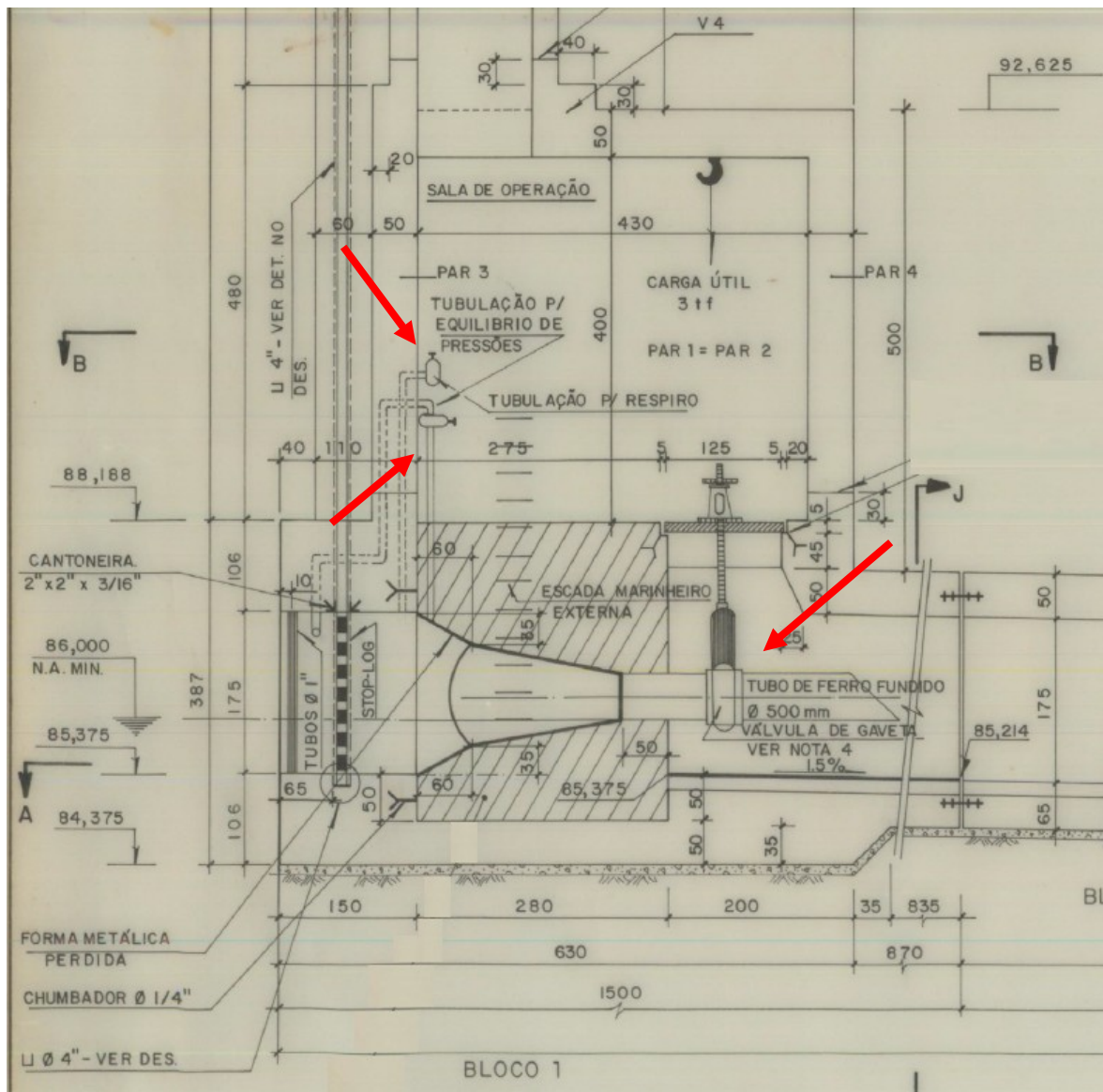
Figura 4 – Detalhe dos equipamentos que serão substituídos na tomada d'água
