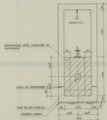
CORTE "II"
