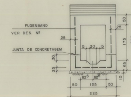
CORTE "GG"
