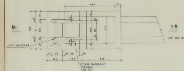
CORTE "CC"
